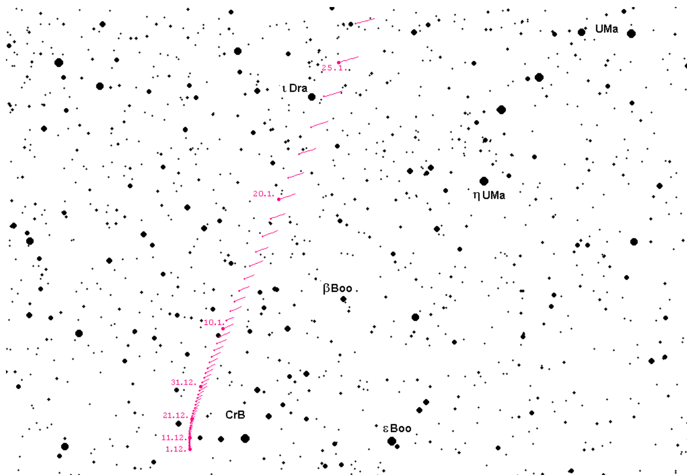
Bewegung des Kometen C/2022 E3 (ZTF) vom 1.12.2022 bis 26.1.2023
